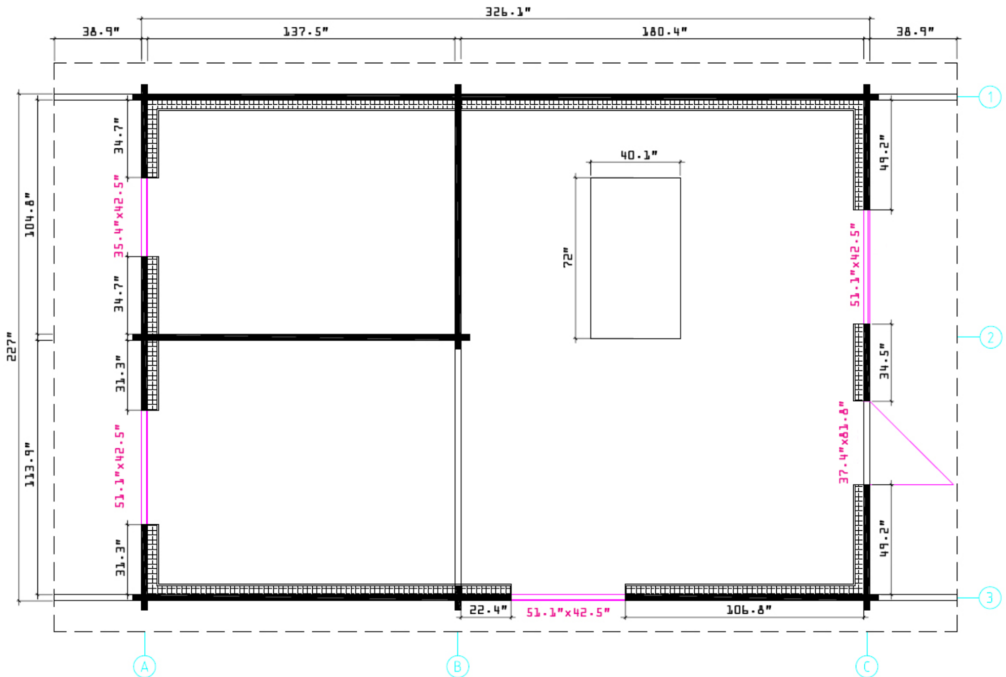
MUSKOKA // 70 / 18 - FLOOR PLAN
