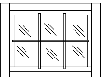
Window 765x990
